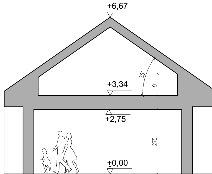
Przekrój
