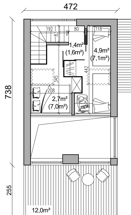
Poddasze
