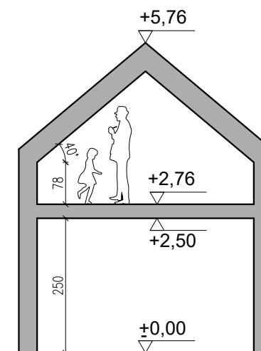
Przekrój
